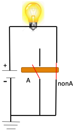
CIRCUITO CON UN INTERRUTTORE INVERTITORE SIMULA LOGIC GATE NOT
