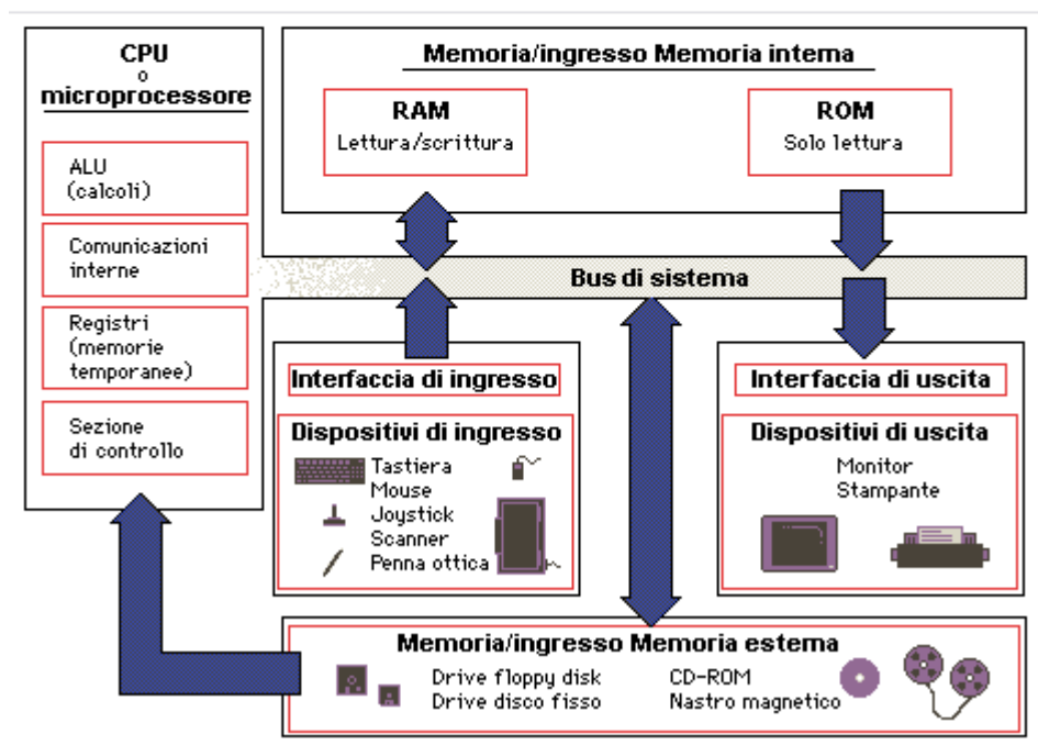
Figura 65 Schema dettagliato di un computer
