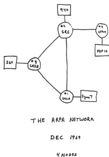
Figura 82 I primi quattro nodi di ARPAnet
