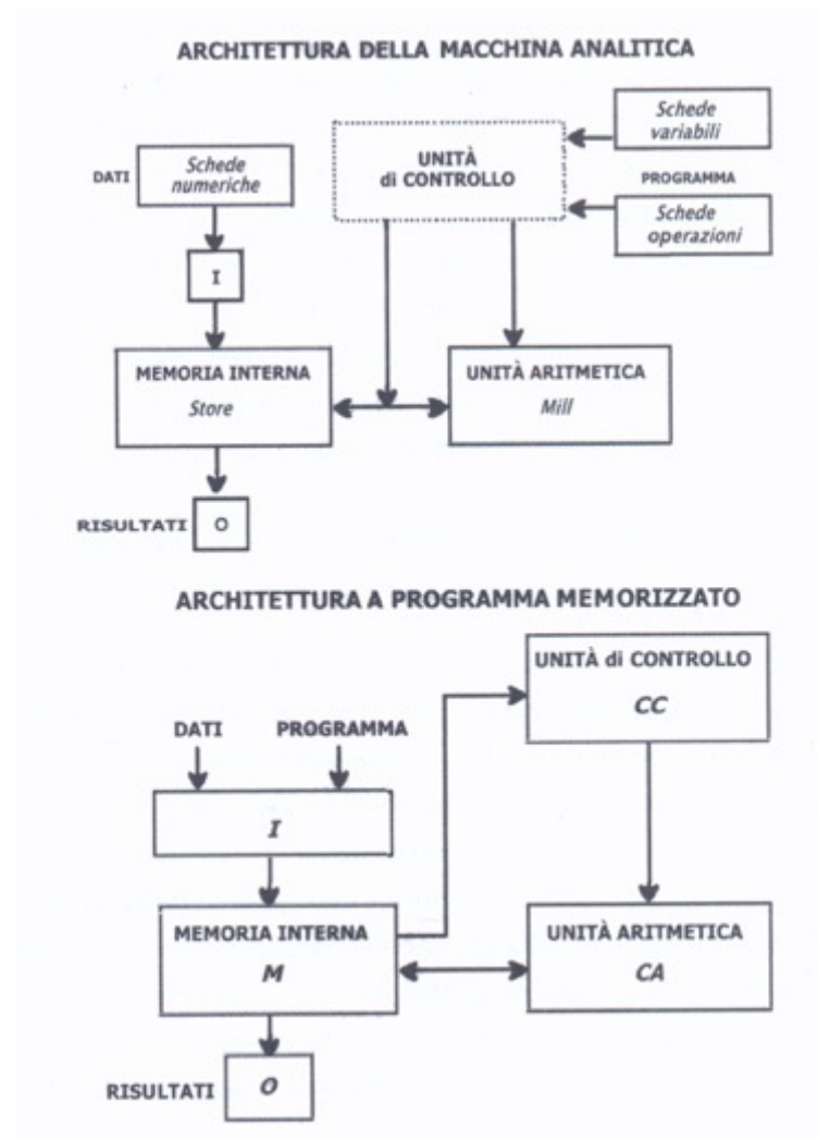
Figura 22 Confronto tra le architetture della "The ANALYTICAL ENGINE" e il moderno computer. O sta per OUTPUT e I sta per INPUT
