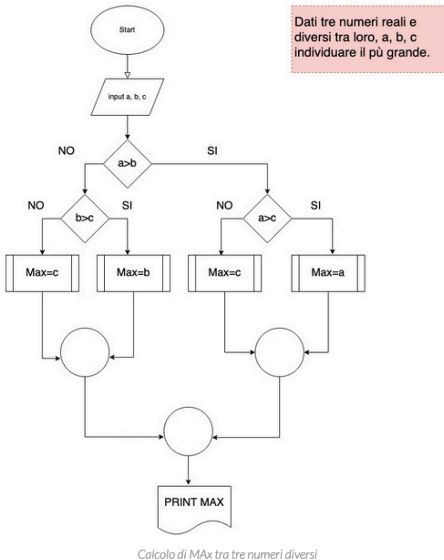
Figura 61 Flow Chart per il calcolo del MAX tra tre numeri
