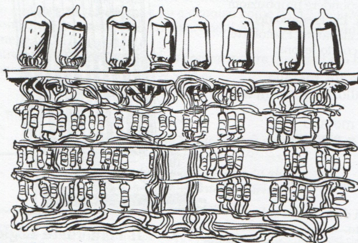
Porte logiche ottenute con diodi e valvole termoioniche, 1952.
