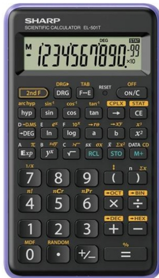
Figura 8 Logaritmi e loro utilizzo con una calcolatrice scientifica
