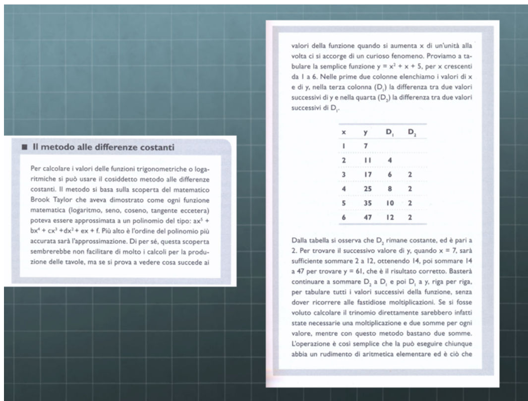
Figura 12 Spiegazione matematica delle differenze costanti 1
