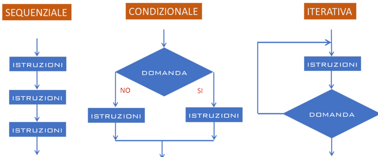
Figura 59 le tre strutture principali per definire e strutturare un algoritmo
