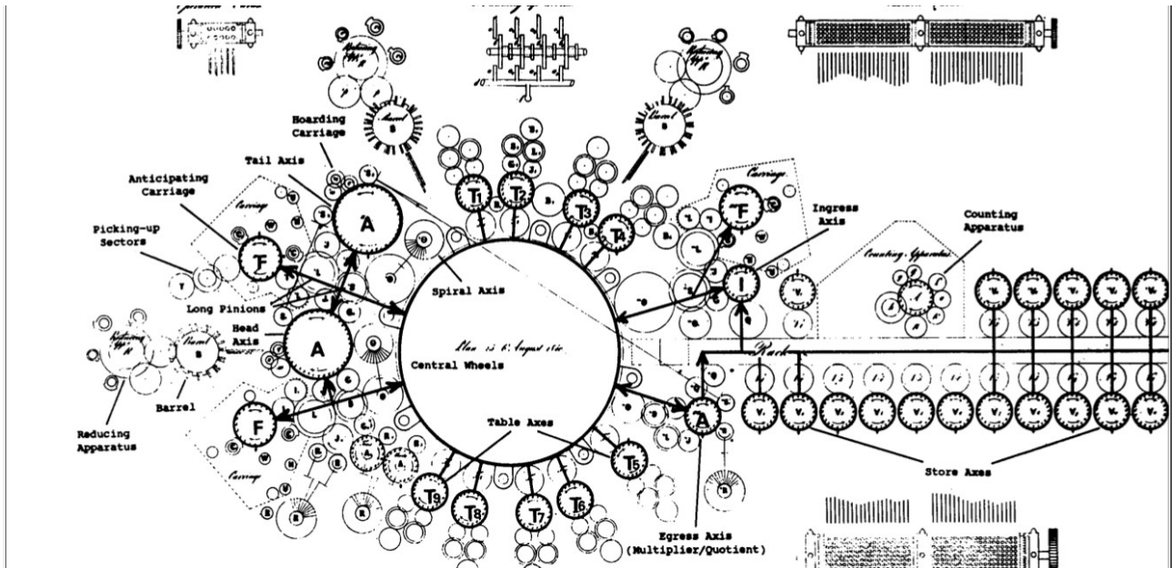
Figura 25 Un parziale schema della "Analytical Engine"
